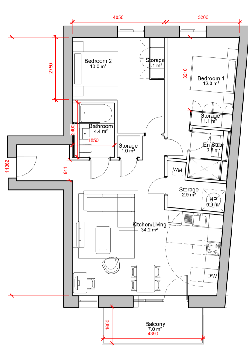
8 2 BED TYPE H 1 : 100
