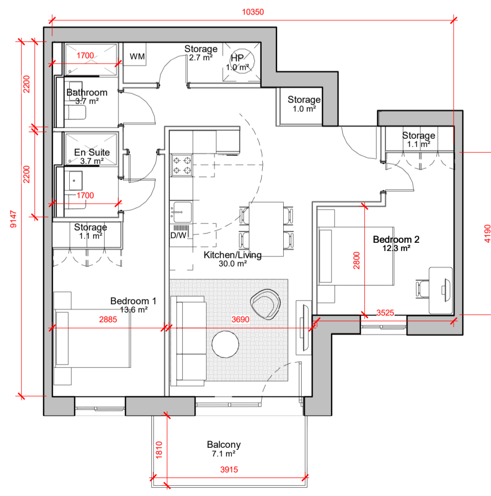
4 2 BED TYPE M 1 : 100
