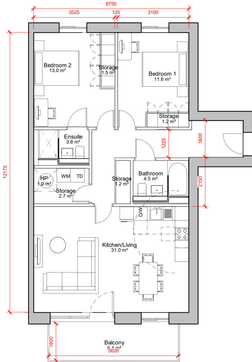
6 2 BED TYPE G 1 : 100
