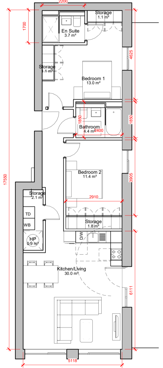
7 2 BED TYPE G2 1 : 100
