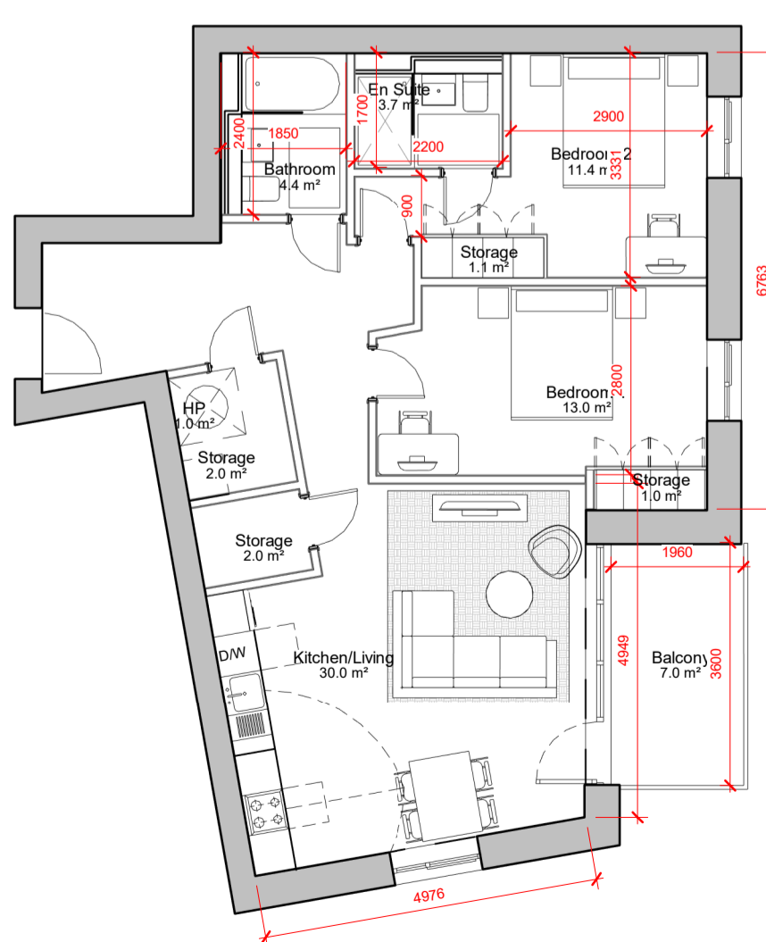
3 2 BED TYPE L 1 : 100
